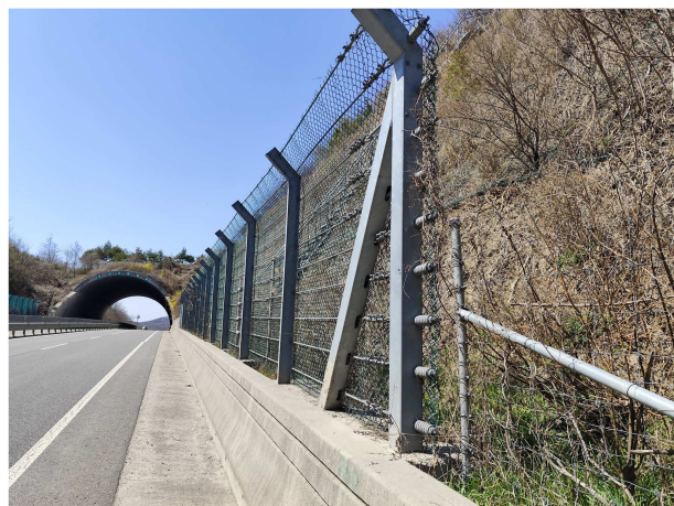
낙석방지울타리 전경
